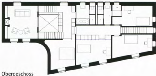
Obergeschoss
