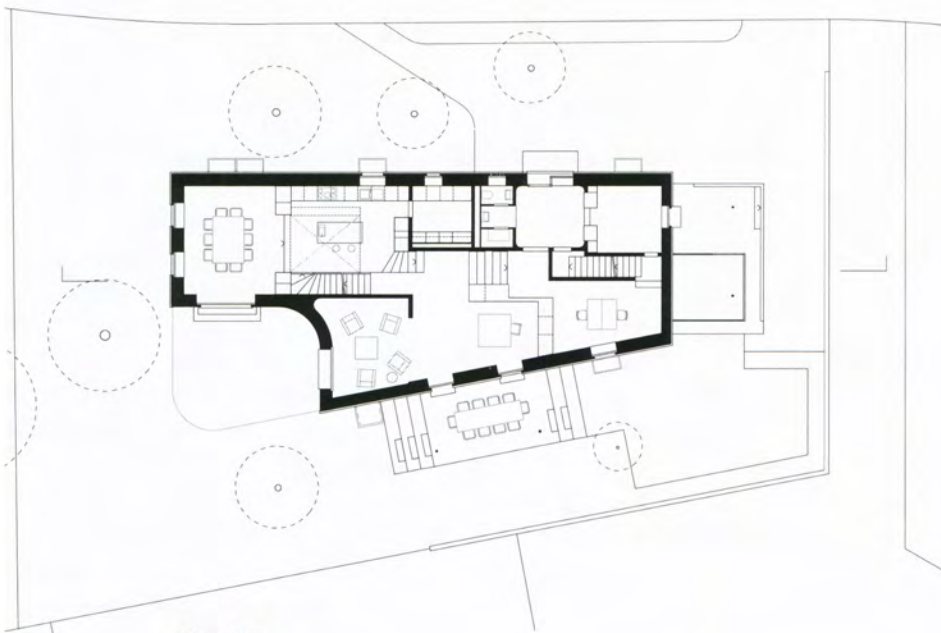
Erdgeschoss
